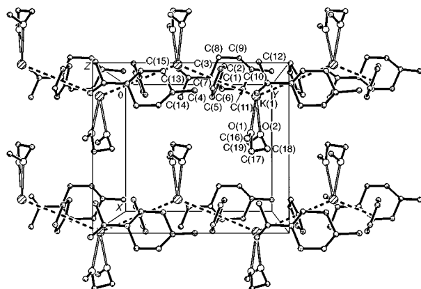
Fig. 4 Unit-cell contents of compound 3c viewed along the b axis. Selected bond distances (Å) and angles (°): K(1)–C(1) 3.194(2), K(1)–C(2) 3.145(1), K(1)–C(3) 3.013(1), K(1)–C(4) 2.979(1), K(1)–C(5) 3.068(1), K(1)–O(1) 2.832(2), K(1)–O(2) 2.923(2), K(1)–C(1a) 3.343(2), K(1)–C(2a) 3.183(1), K(1)–C(3a) 2.980(1), K(1)–C(4a) 2.982(1) and K(1)–C(5a) 3.200(1); C(1)–K(1)–C(2) 25.7(1), C(1)–K(1)–C(3) 43.4(1), C(2)–K(1)–C(3) 26.4(1), C(1)–K(1)–C(4) 43.5(1), C(2)–K(1)–C(4) 43.1(1), C(3)–K(1)–C(4) 26.8(1), C(1)–K(1)–C(5) 25.9(1), C(2)–K(1)–C(5) 42.2(1), C(3)–K(1)–C(5) 43.3(1), C(4)–K(1)–C(5) 26.5(1) and O(1)–K(1)–O(2) 59.0(1)
